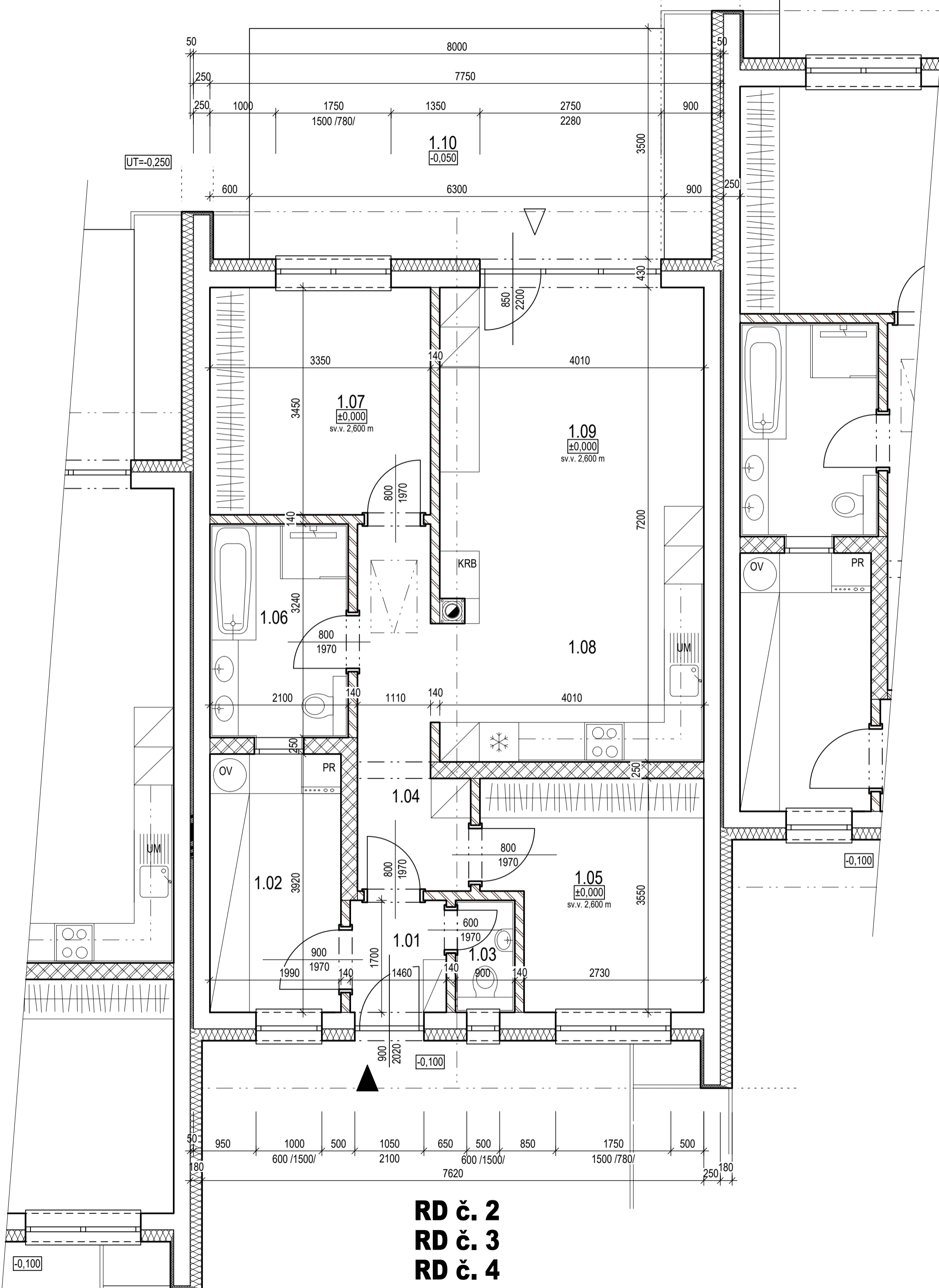
PÔDORYS 1.N.P. M1:50
