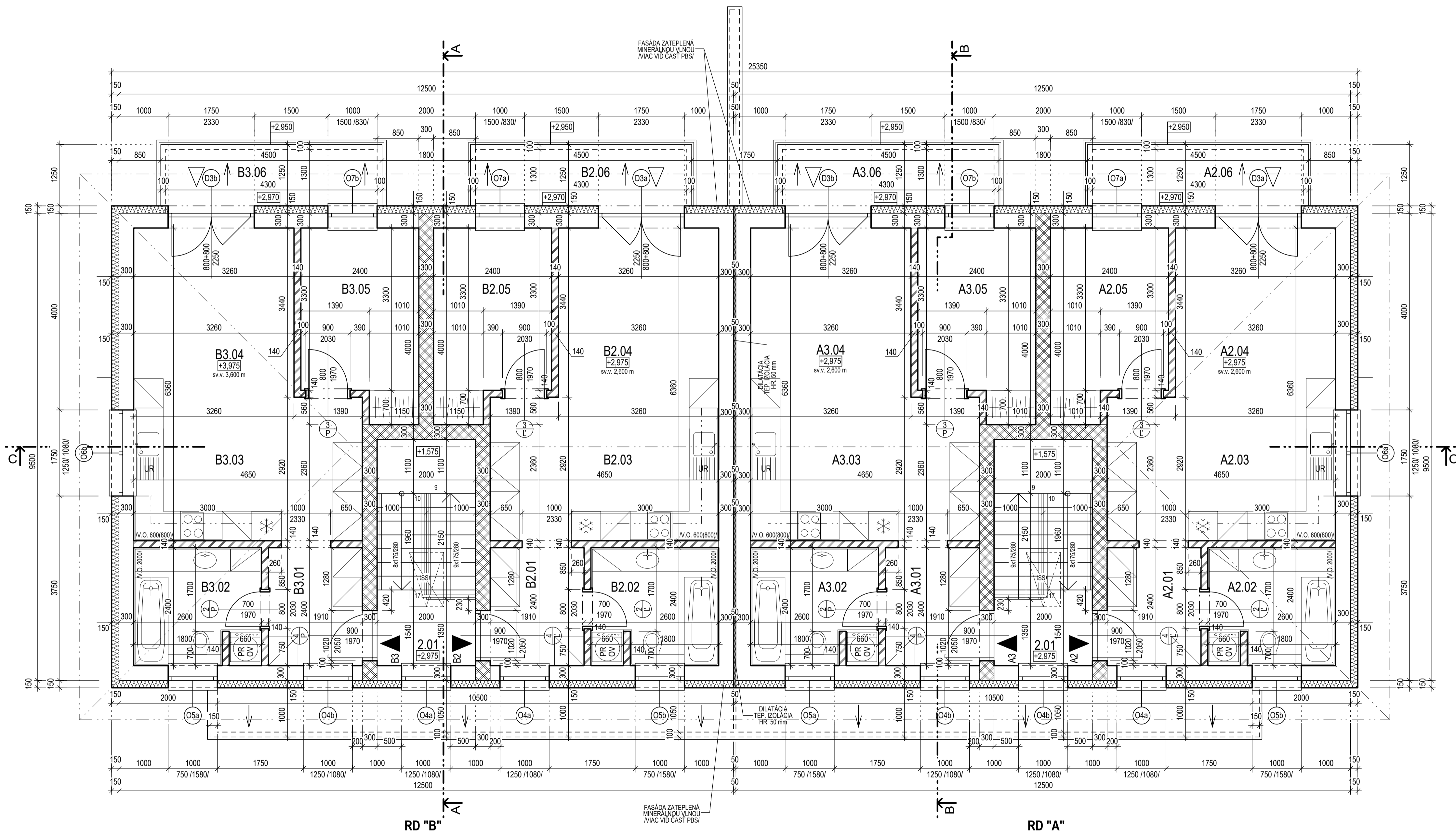
PÓDORYS 2.N.P. M1:50
