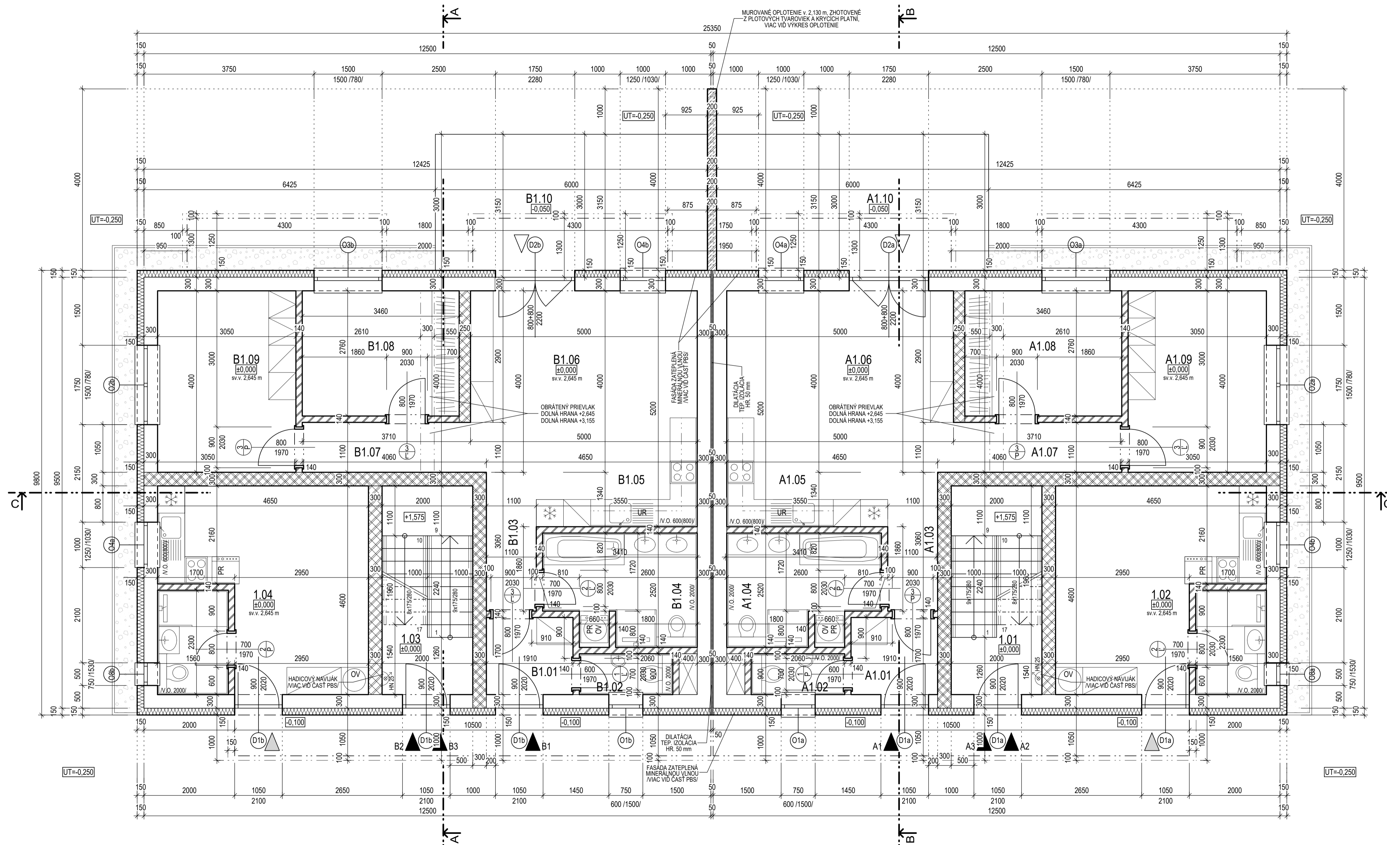
PÔDORYS 1.N.P. M1:50
