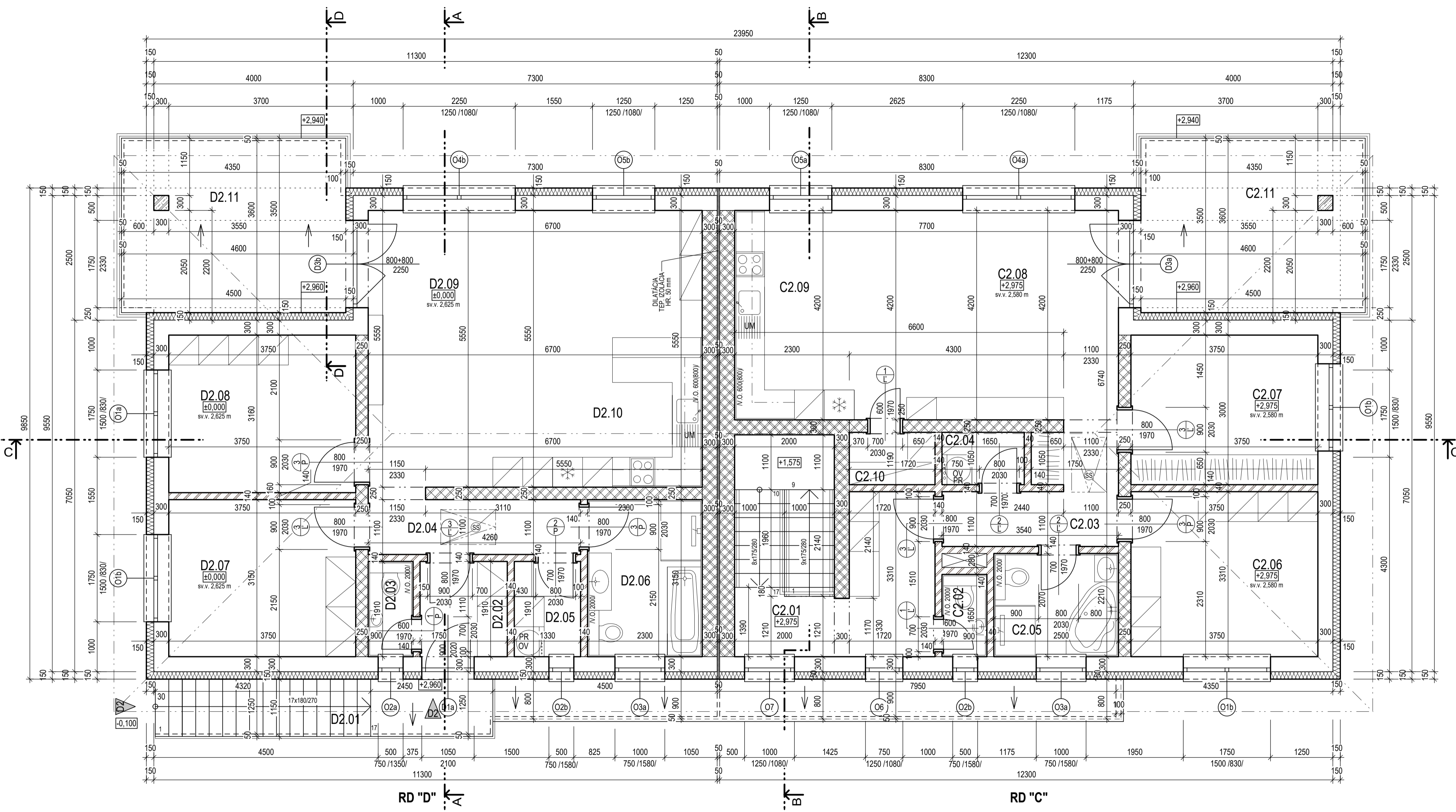
PÔDORYS 2.N.P. M1:50
