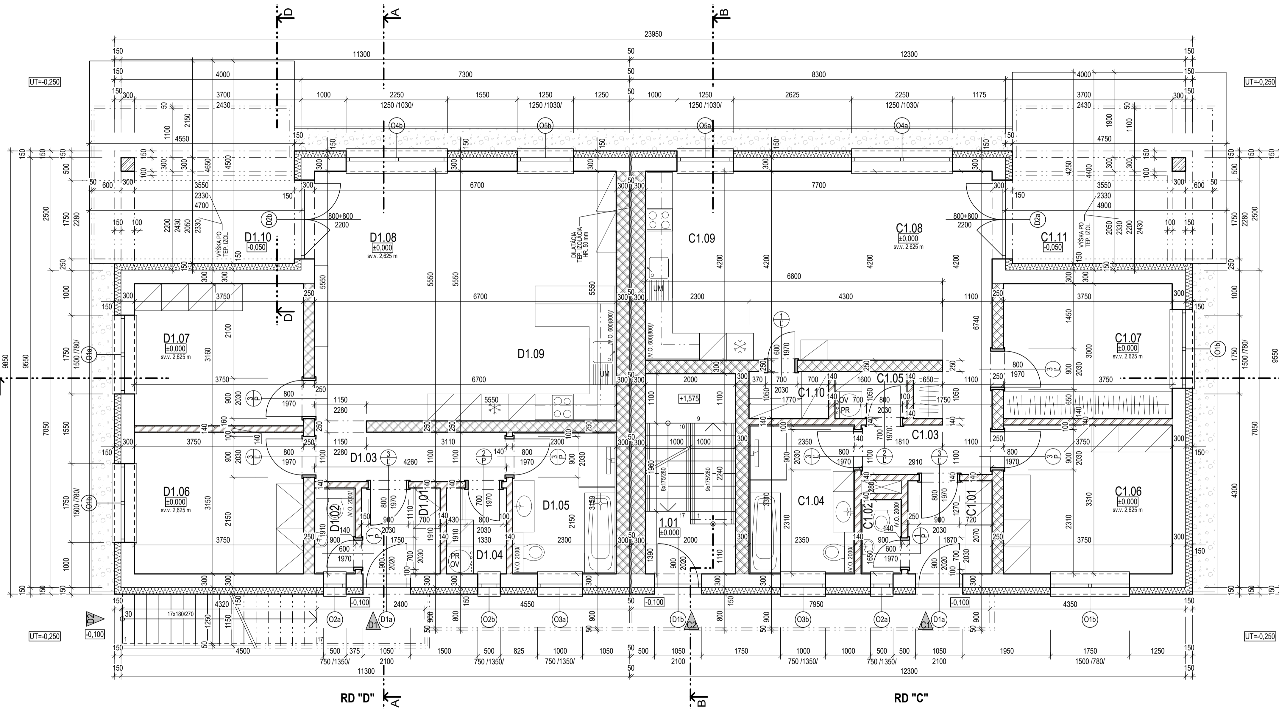
PÔDORYS 1.N.P. M1:50
